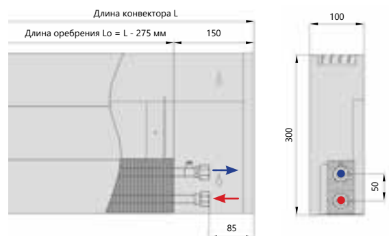
Боковое подключение
