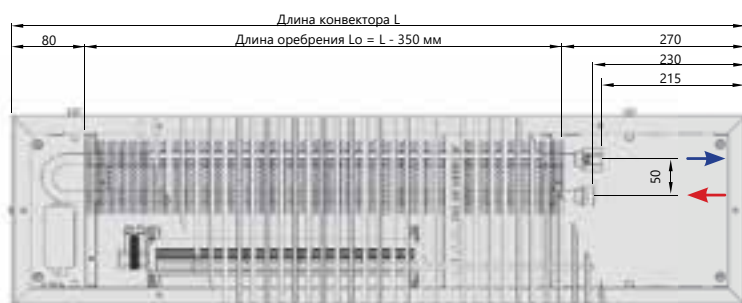
Вид сверху
