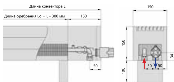
Нижнее подключение
