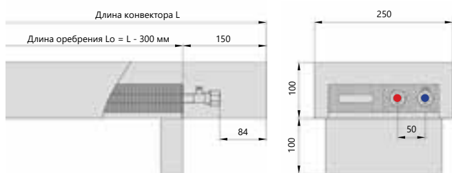
Боковое подключение
