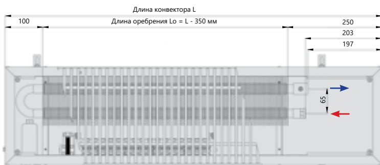
Вид сверху
