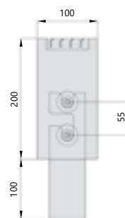
Поперечный разрез
