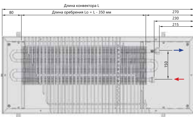
Вид сверху
