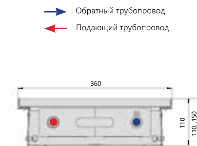
Поперечный разрез
