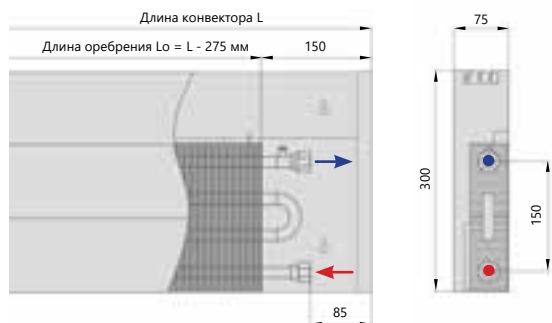
Боковое подключение
