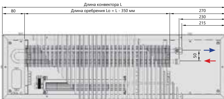
Вид сверху
