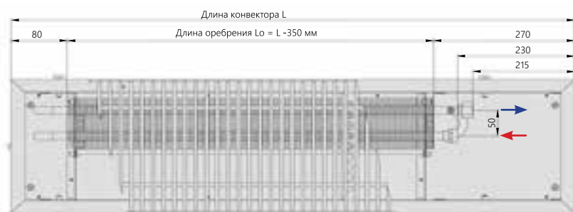
Вид сверху
