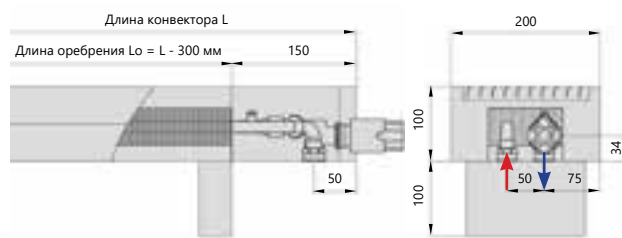
Нижнее подключение
