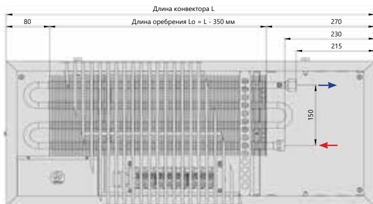
Вид сверху
