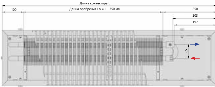
Вид сверху
