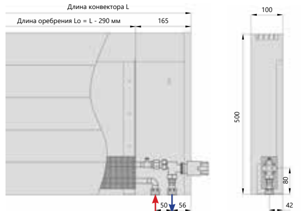
Нижнее подключение
