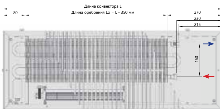
Вид сверху
