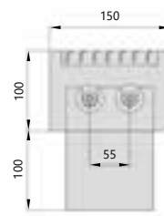
Поперечный разрез
