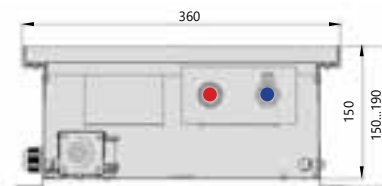
Поперечный разрез
