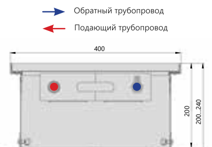
Поперечный разрез
