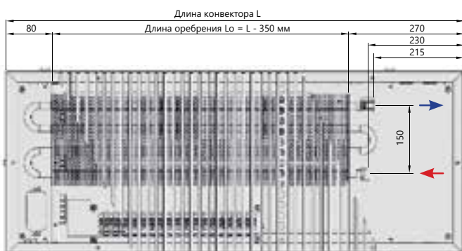
Вид сверху
