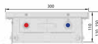
Поперечный разрез
