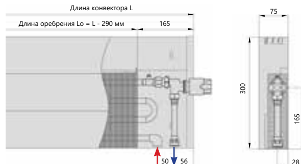
Нижнее подключение
