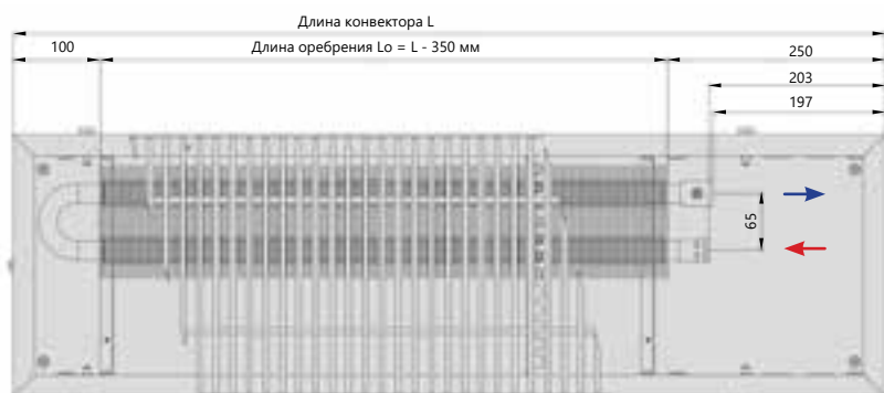
Вид сверху
