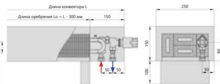
Нижнее подключение
