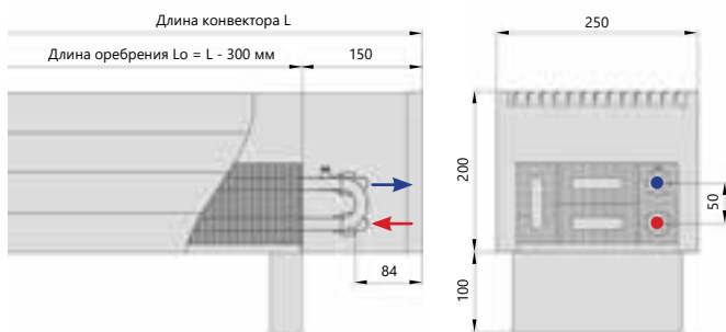
Боковое подключение
