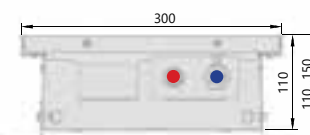
Поперечный разрез
