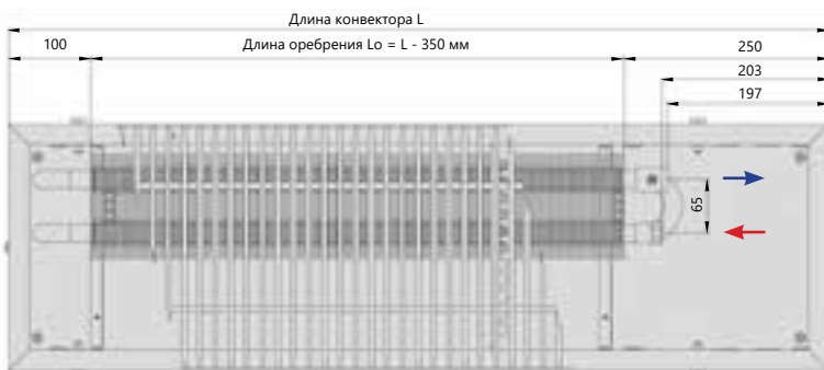
Вид сверху
