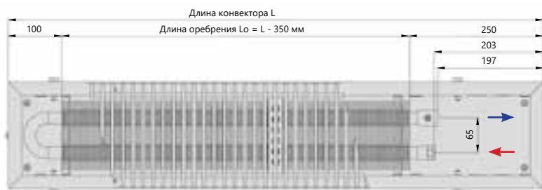
Вид сверху
