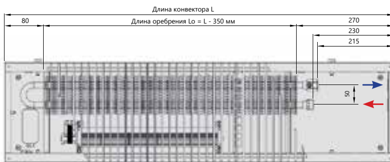
Вид сверху
