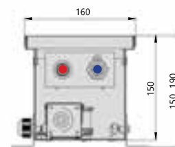
Поперечный разрез
