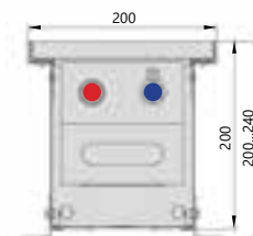
Поперечный разрез
