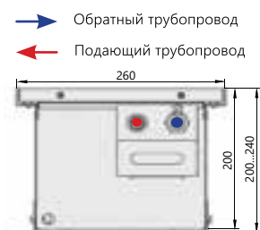
Поперечный разрез
