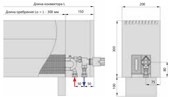
Нижнее подключение
