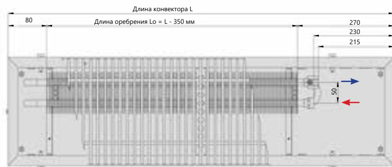
Вид сверху
