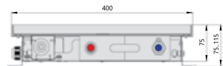
Поперечный разрез
