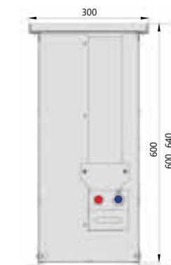
Поперечный разрез
