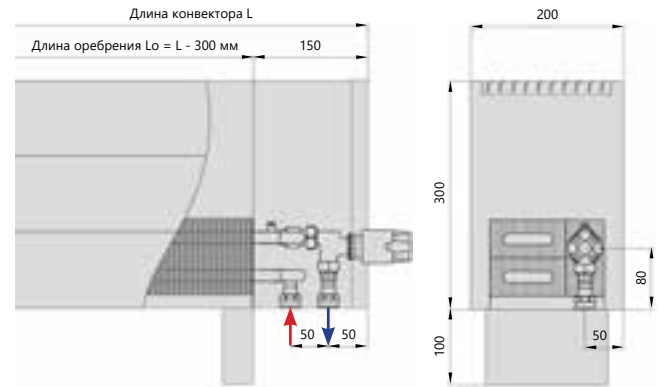
Нижнее подключение
