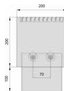
Поперечный разрез
