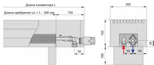
Нижнее подключение
