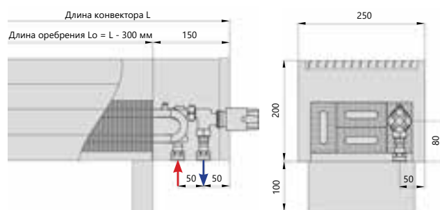
Нижнее подключение
