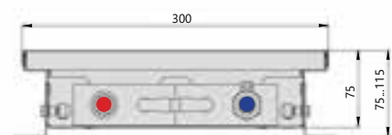
Поперечный разрез
