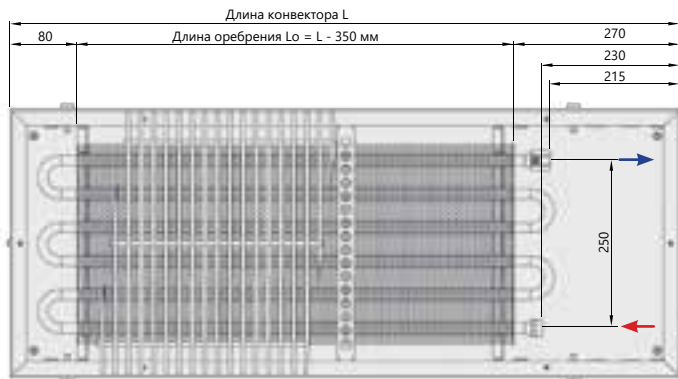
Вид сверху
