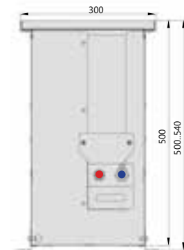
Поперечный разрез
