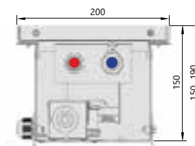
Поперечный разрез
