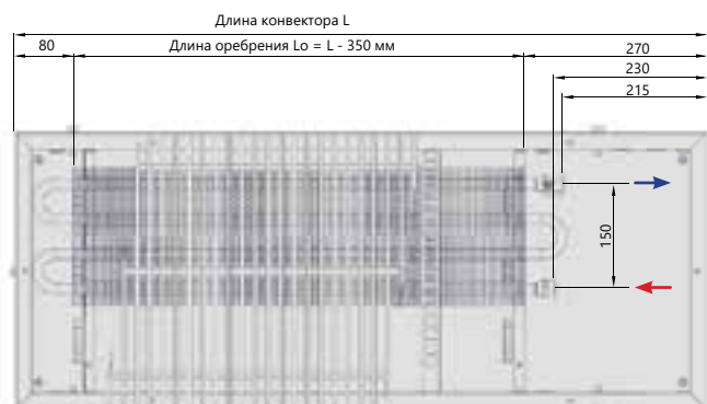
Вид сверху
