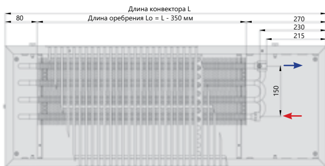
Вид сверху
