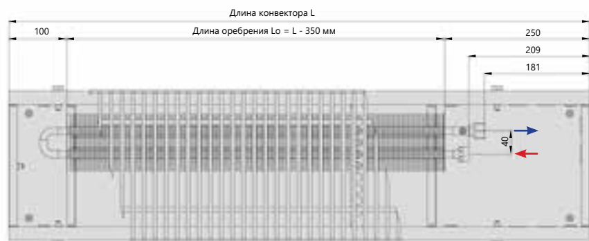
Вид сверху
