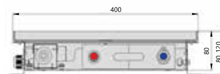
Поперечный разрез
