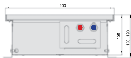
Поперечный разрез
