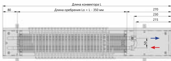
Вид сверху
