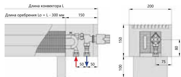
Нижнее подключение
