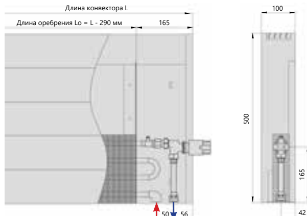
Нижнее подключение
