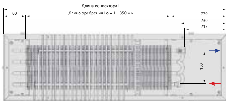
Вид сверху
