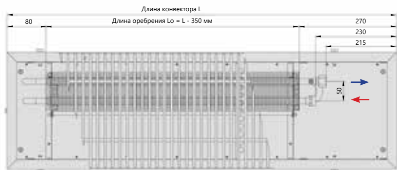
Вид сверху
