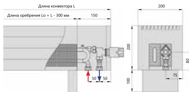
Нижнее подключение
