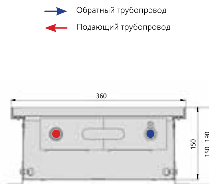
Поперечный разрез
