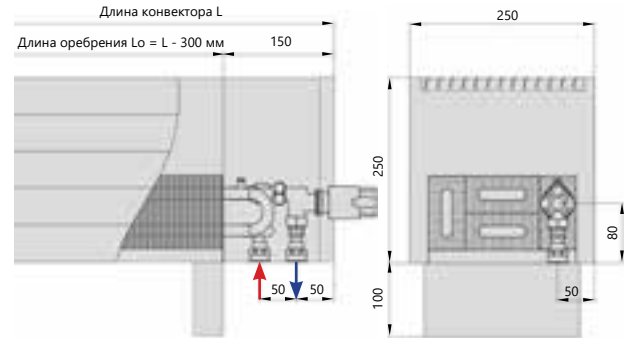
Нижнее подключение
