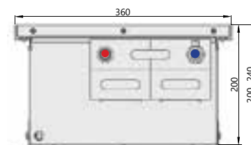
Поперечный разрез
