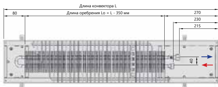
Вид сверху
