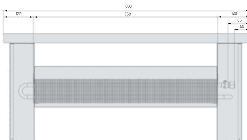
Вид спереди
