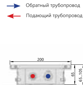
Поперечный разрез
