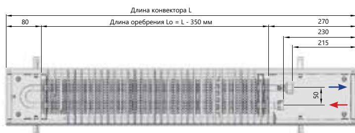
Вид сверху
