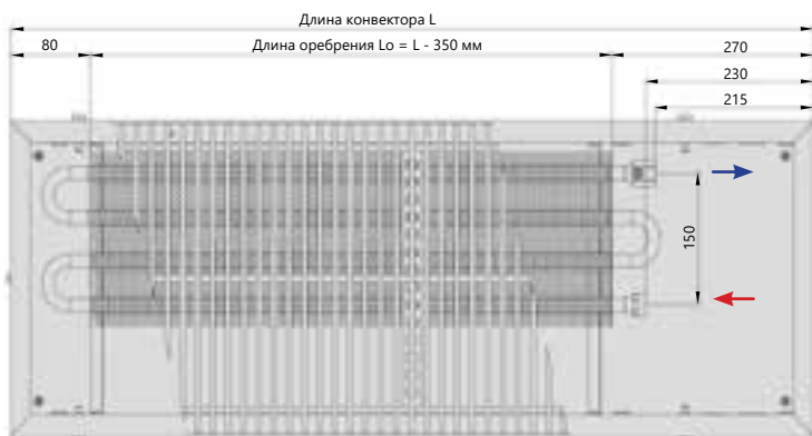
Вид сверху
