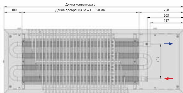
Вид сверху
