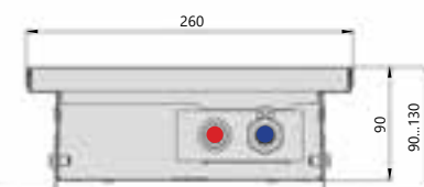
Поперечный разрез
