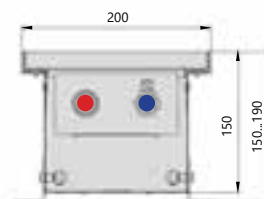
Поперечный разрез
