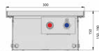
Поперечный разрез
