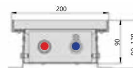
Поперечный разрез
