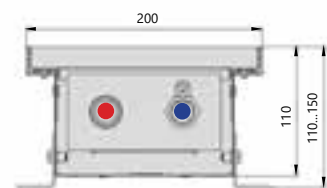
Поперечный разрез
