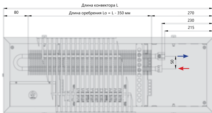
Вид сверху
