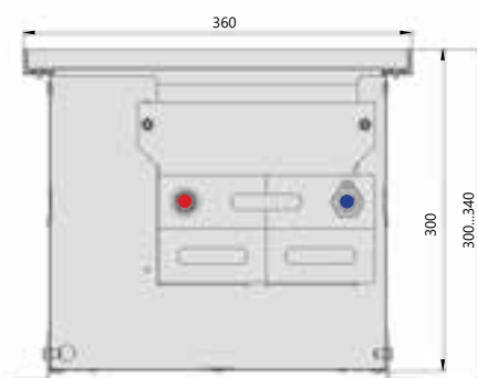
Поперечный разрез
