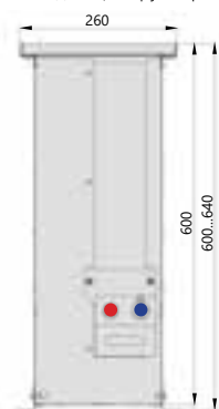
Поперечный разрез
