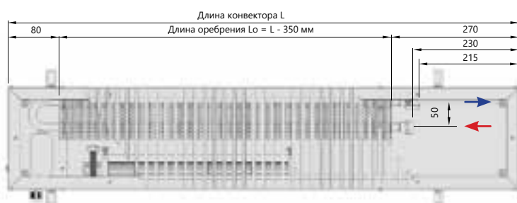
Вид сверху
