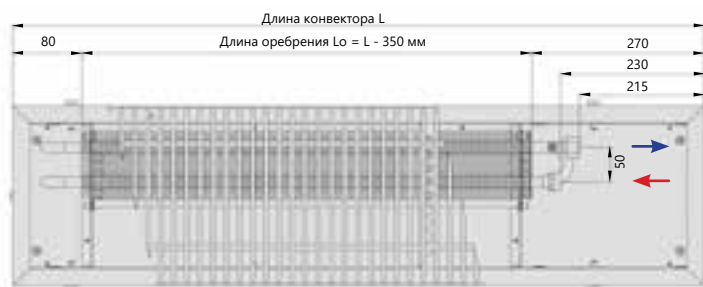
Вид сверху
