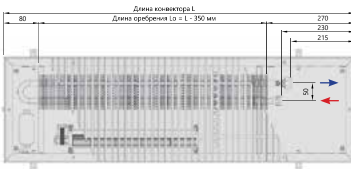
Вид сверху
