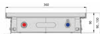
Поперечный разрез
