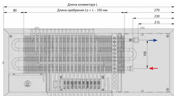
Вид сверху
