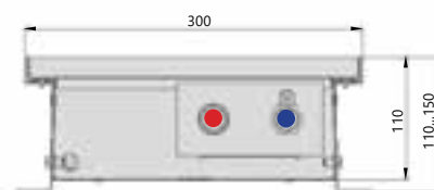
Поперечный разрез
