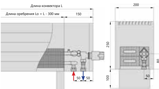
Нижнее подключение
