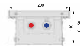
Поперечный разрез
