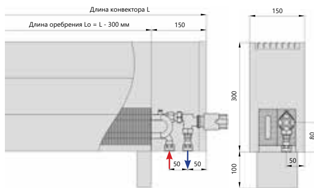
Нижнее подключение
