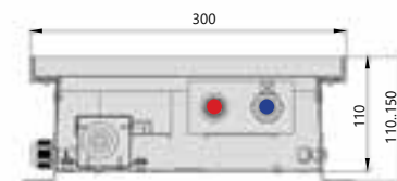
Поперечный разрез
