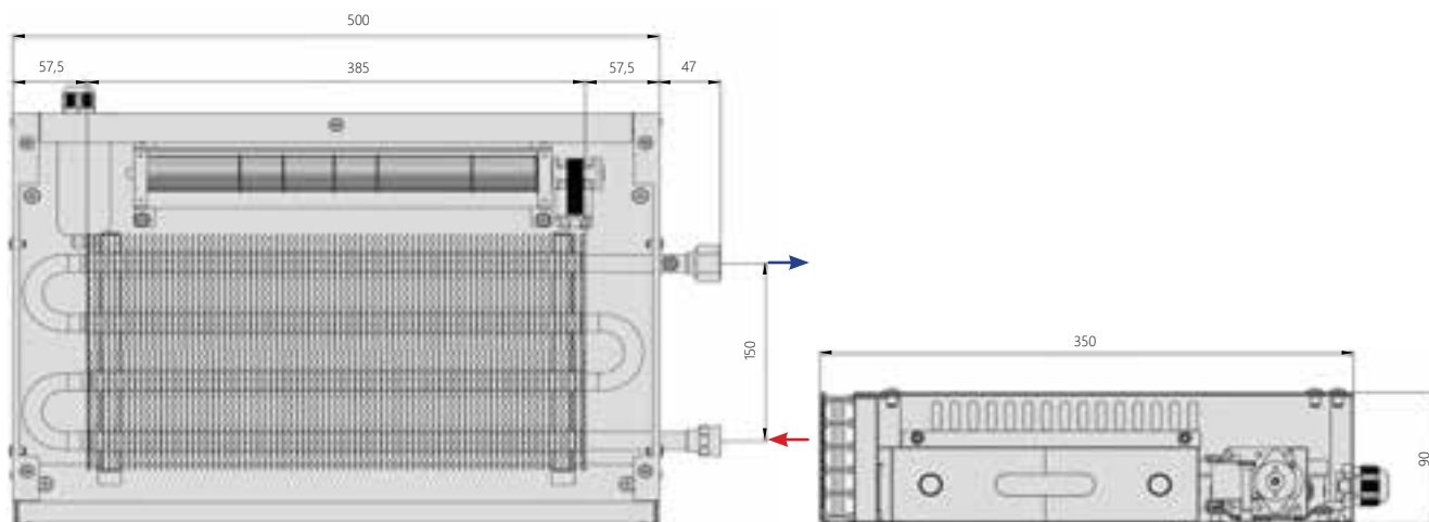
Вид сверху
