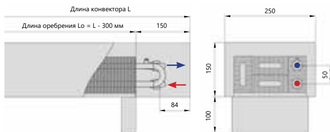
Боковое подключение
