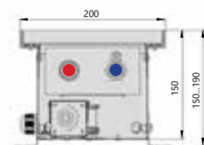
Поперечный разрез
