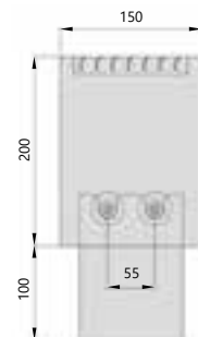
Поперечный разрез
