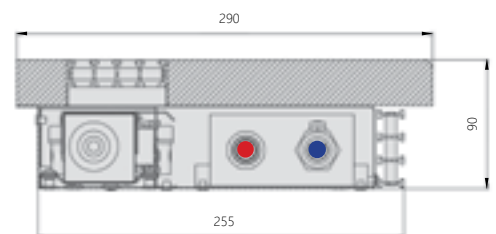
Поперечный разрез
