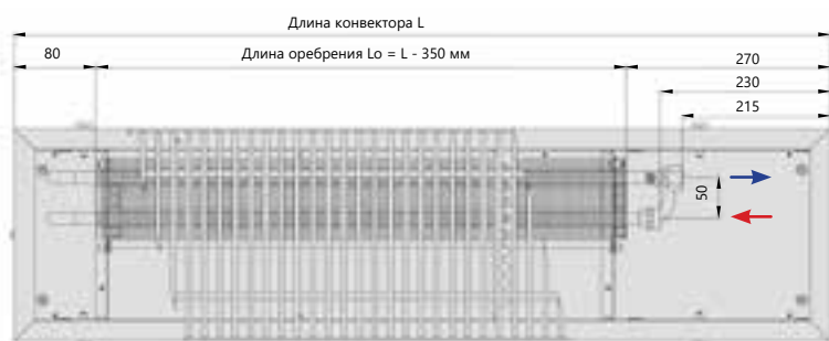
Вид сверху
