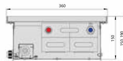
Поперечный разрез
