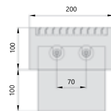
Поперечный разрез
