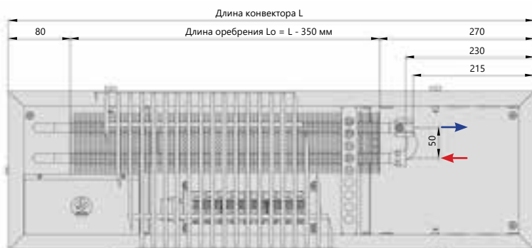
Вид сверху
