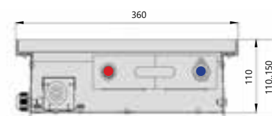
Поперечный разрез
