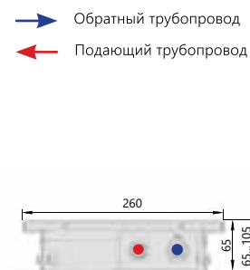
Поперечный разрез
