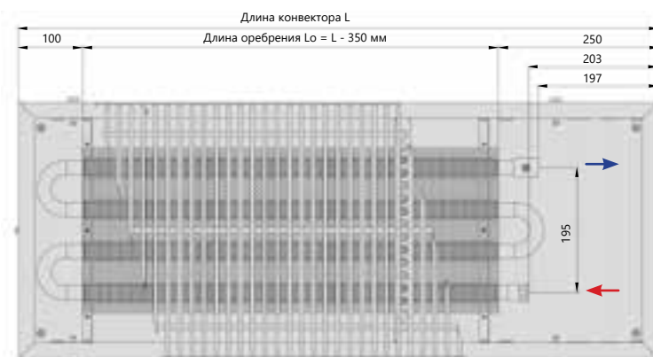
Вид сверху
