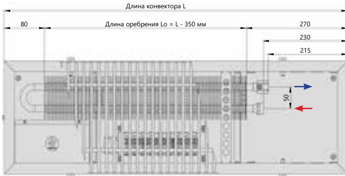
Вид сверху
