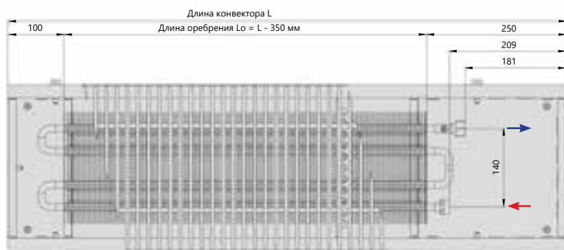
Вид сверху
