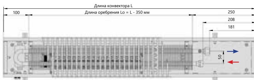
Вид сверху
