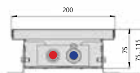
Поперечный разрез
