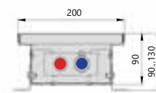
Поперечный разрез
