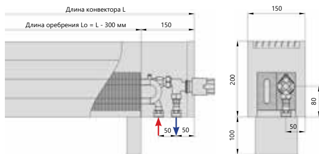
Нижнее подключение
