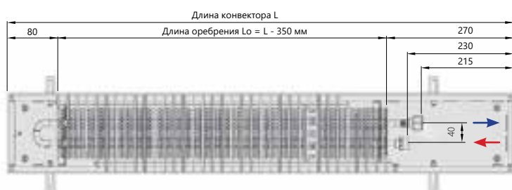
Вид сверху
