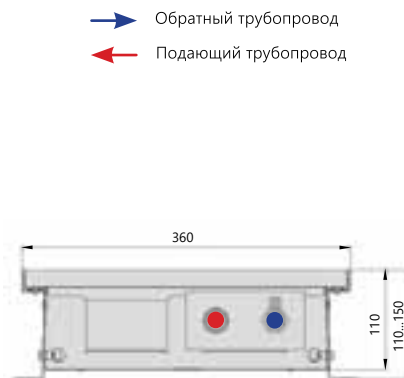
Поперечный разрез
