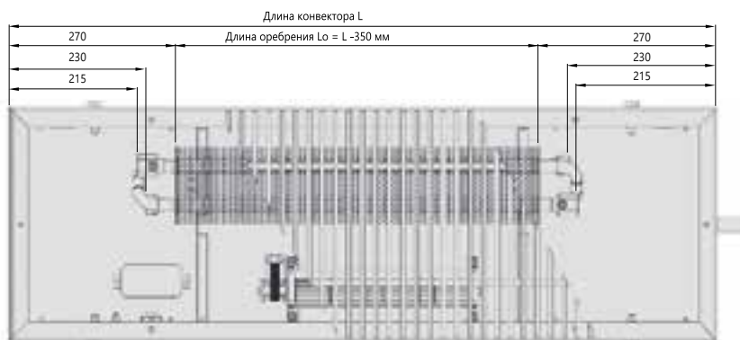
Вид сверху
