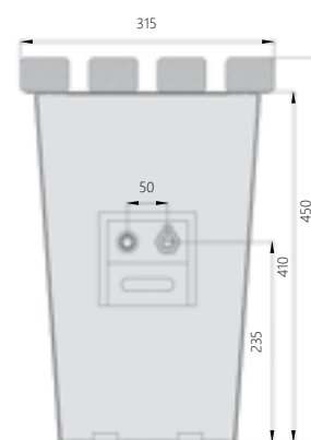
Поперечный разрез
