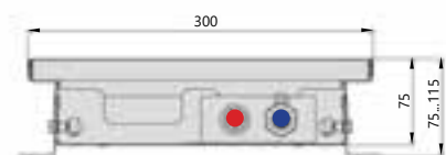
Поперечный разрез
