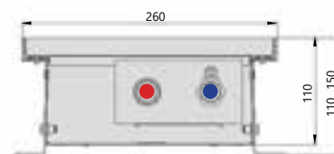
Поперечный разрез
