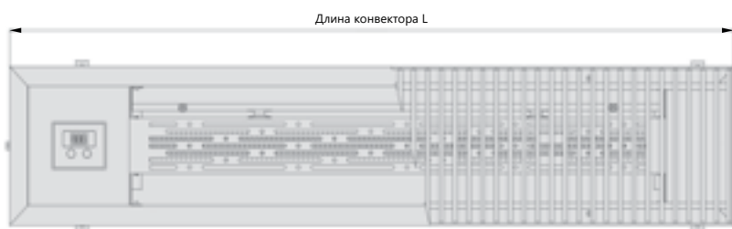
Вид сверху
