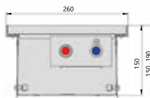
Поперечный разрез
