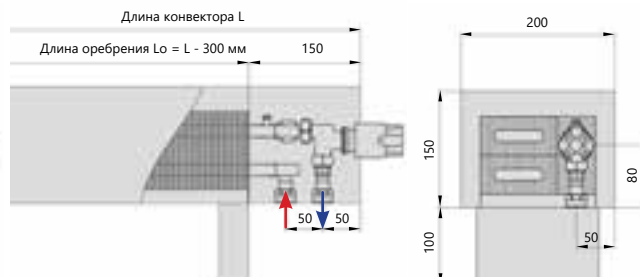
Нижнее подключение
