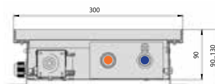
Поперечный разрез
