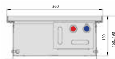
Поперечный разрез
