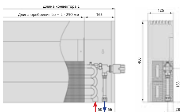
Нижнее подключение
