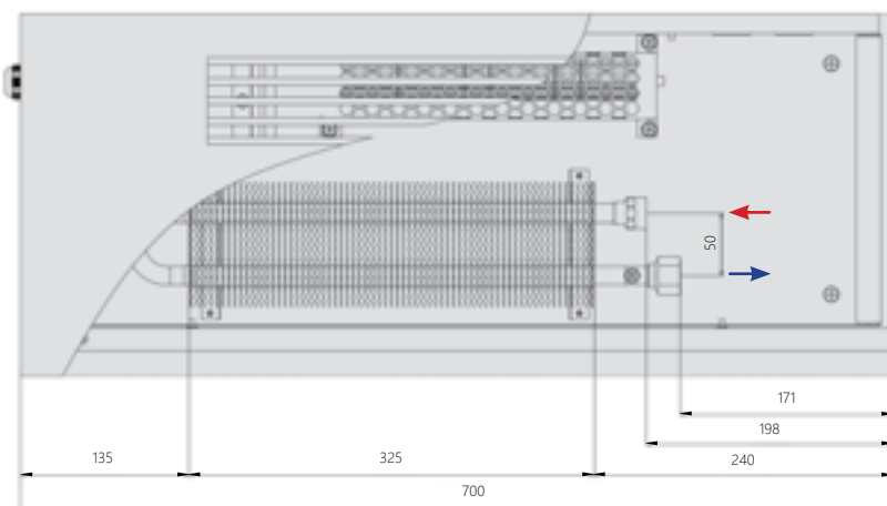
Вид сверху
