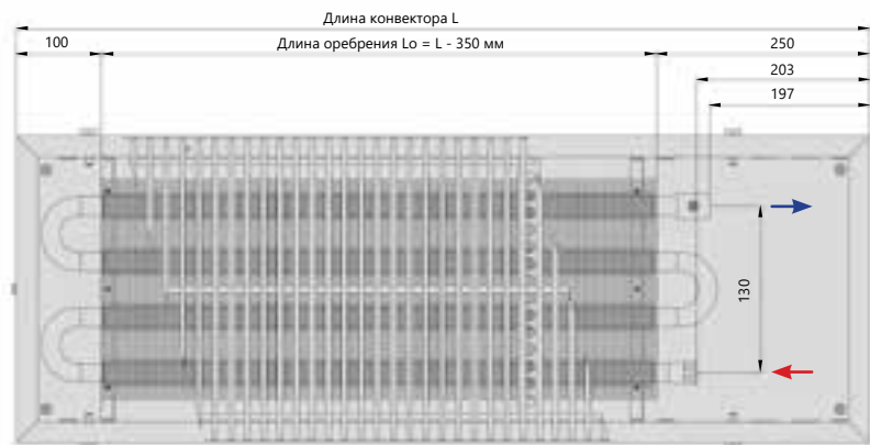
Вид сверху
