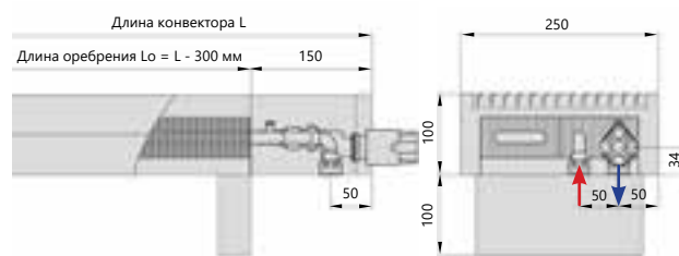
Нижнее подключение
