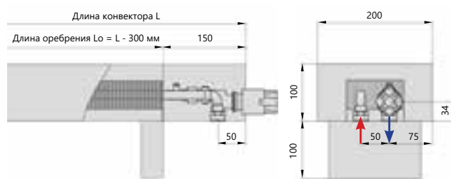
Нижнее подключение
