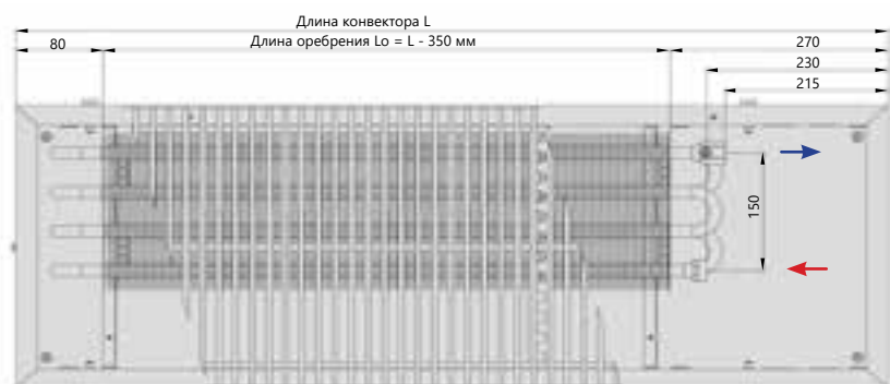
Вид сверху
