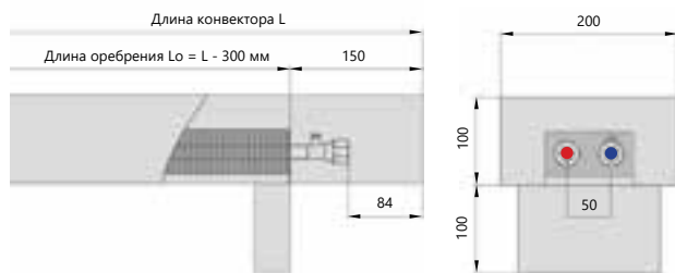
Боковое подключение
