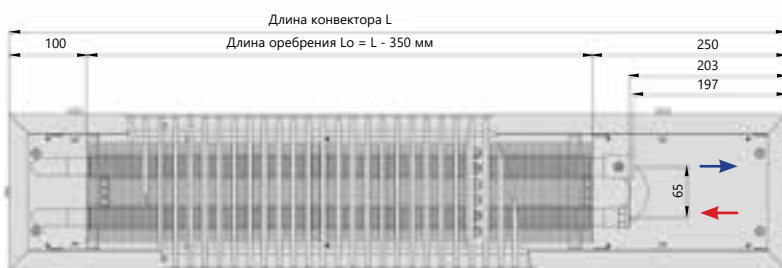
Вид сверху
