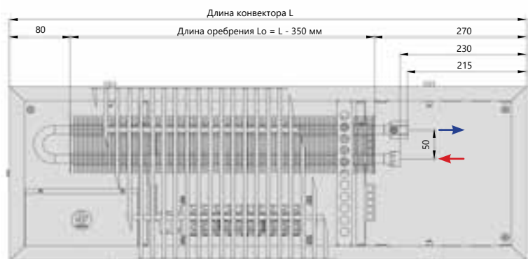
Вид сверху
