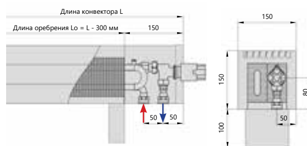
Нижнее подключение
