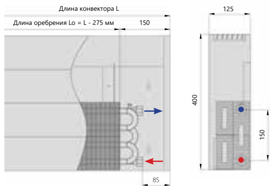
Боковое подключение
