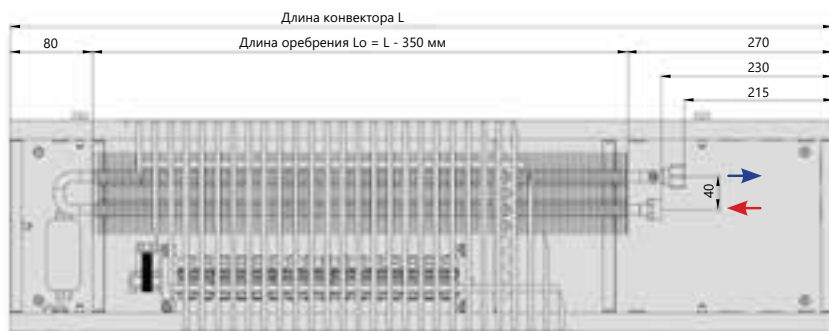
Вид сверху
