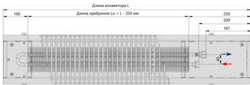
Вид сверху
