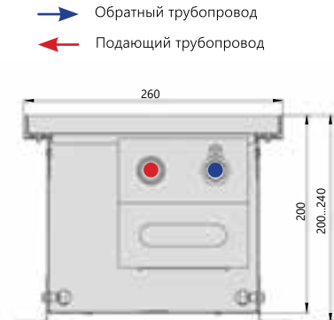
Поперечный разрез
