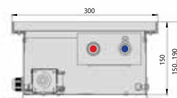
Поперечный разрез
