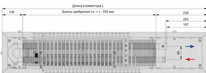
Вид сверху
