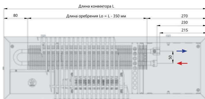
Вид сверху
