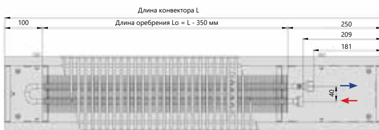
Вид сверху
