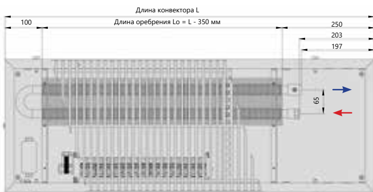
Вид сверху
