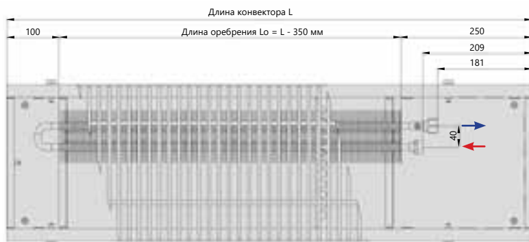
Вид сверху
