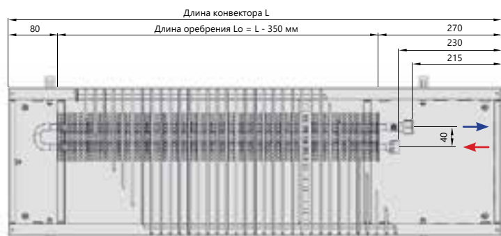
Вид сверху
