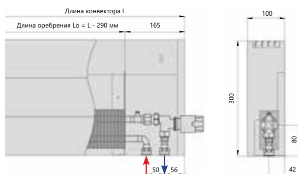
Нижнее подключение
