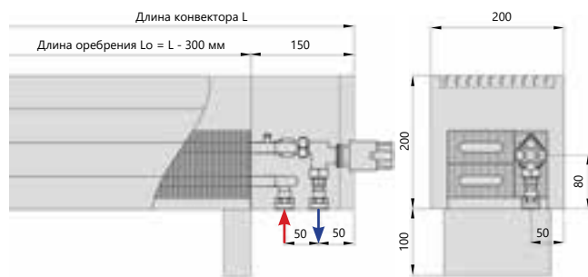
Нижнее подключение
