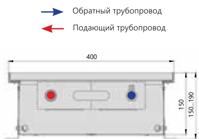
Поперечный разрез
