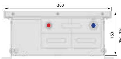
Поперечный разрез
