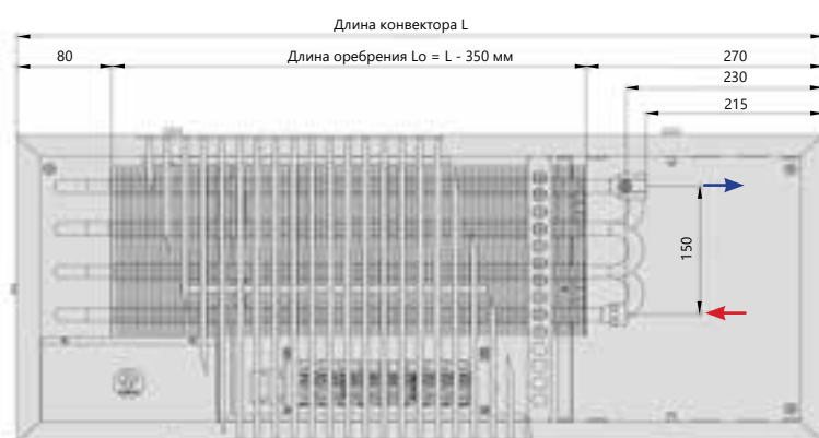
Вид сверху
