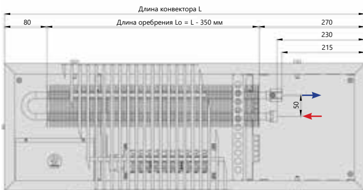
Вид сверху
