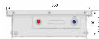
Поперечный разрез
