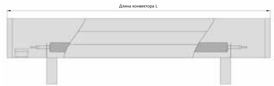
Вид спереди
