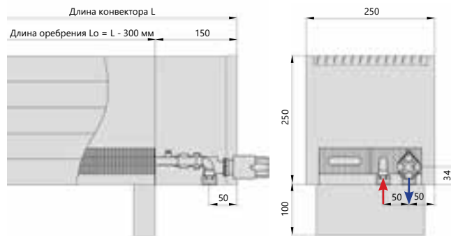
Нижнее подключение
