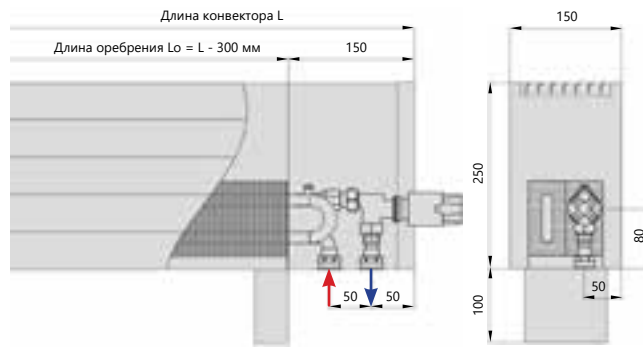
Нижнее подключение
