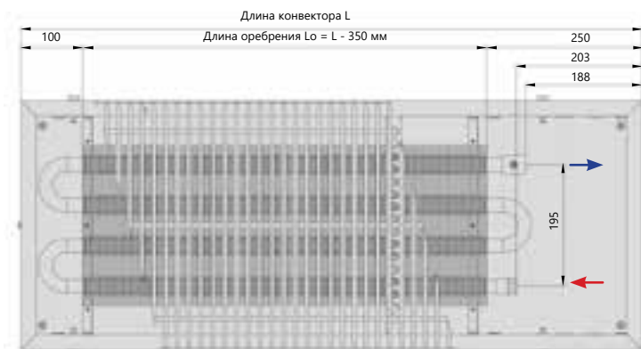
Вид сверху
