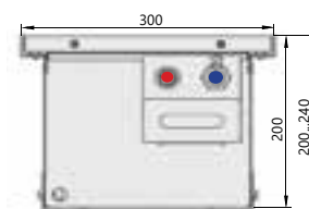
Поперечный разрез
