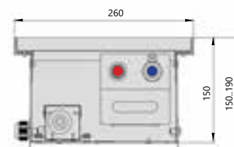
Поперечный разрез
