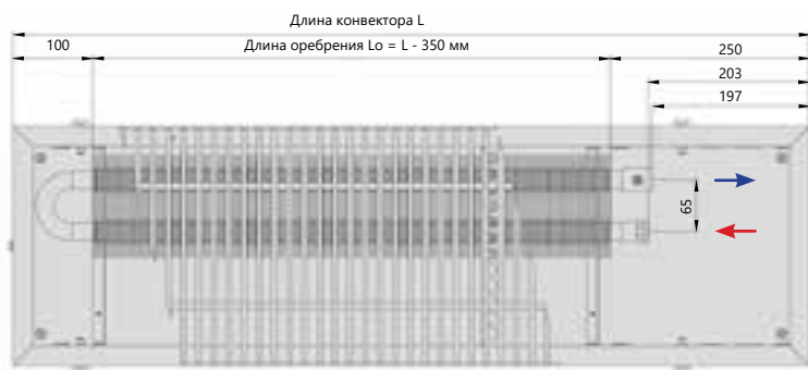
Вид сверху
