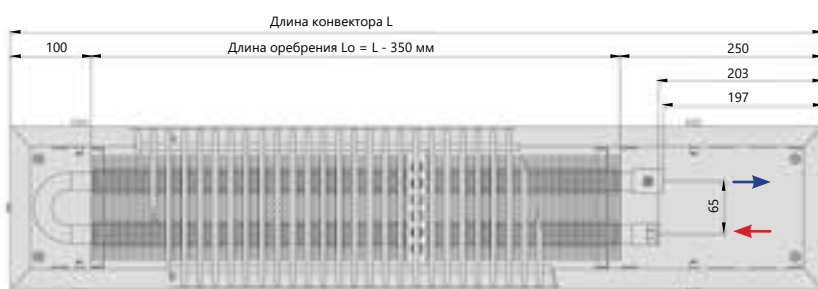
Вид сверху
