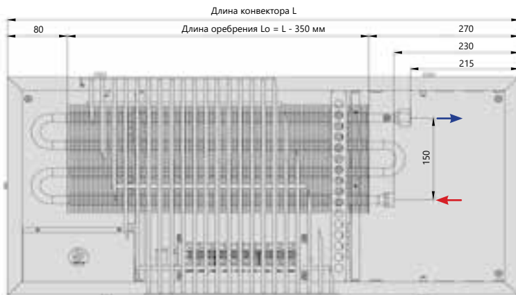
Вид сверху
