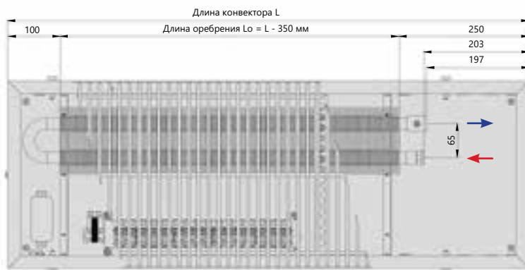
Вид сверху
