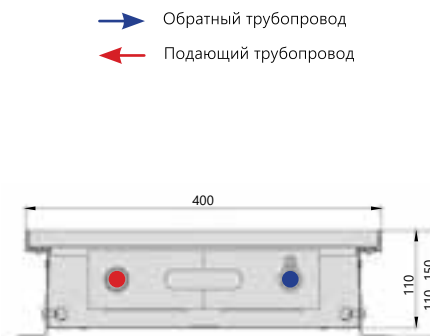
Поперечный разрез
