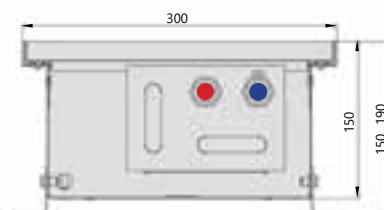
Поперечный разрез
