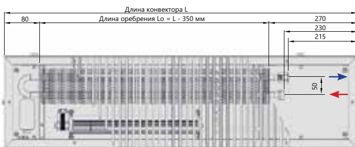
Вид сверху
