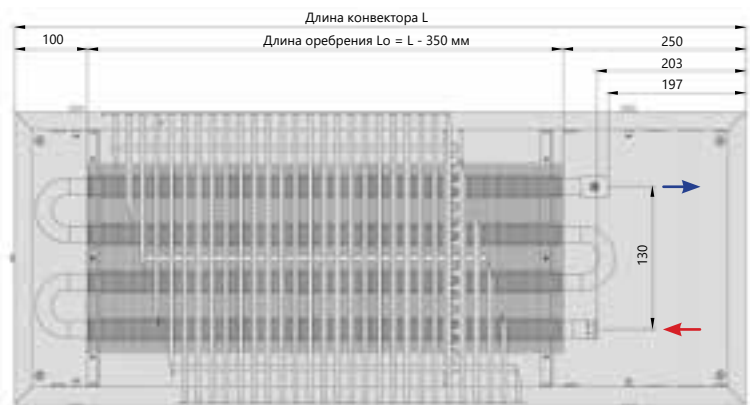
Вид сверху
