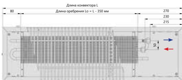
Вид сверху
