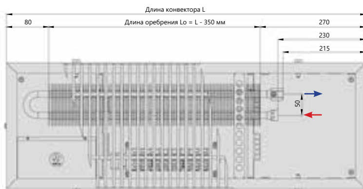
Вид сверху
