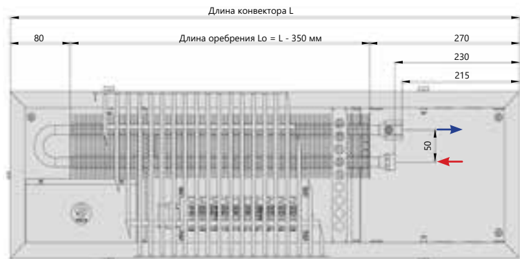
Вид сверху
