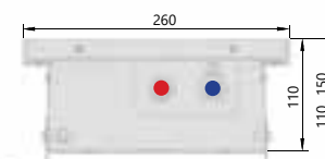
Поперечный разрез
