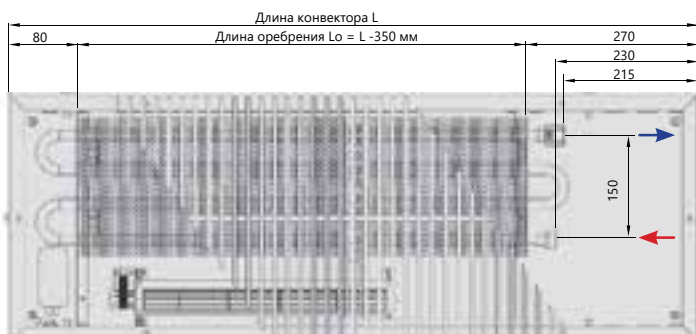
Вид сверху
